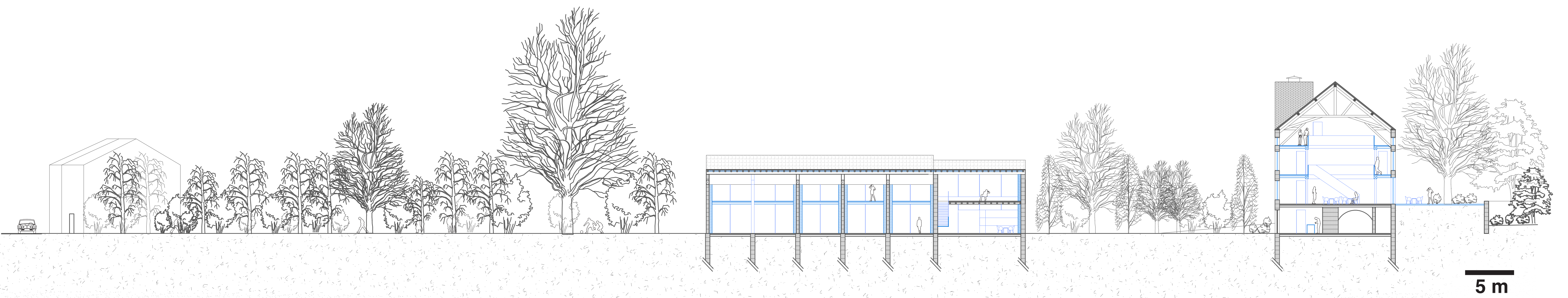
Coupe longitudinale : locaux d'entreprises et brasserie, 1:200
