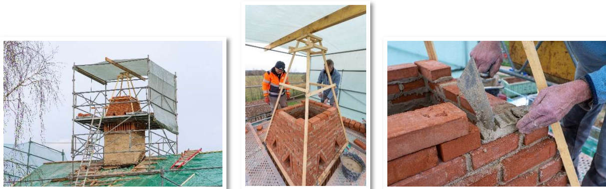
Figure 3 - Réfection de la souche de cheminée
