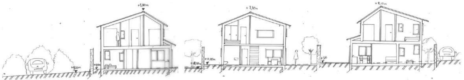
Coupe BB'
