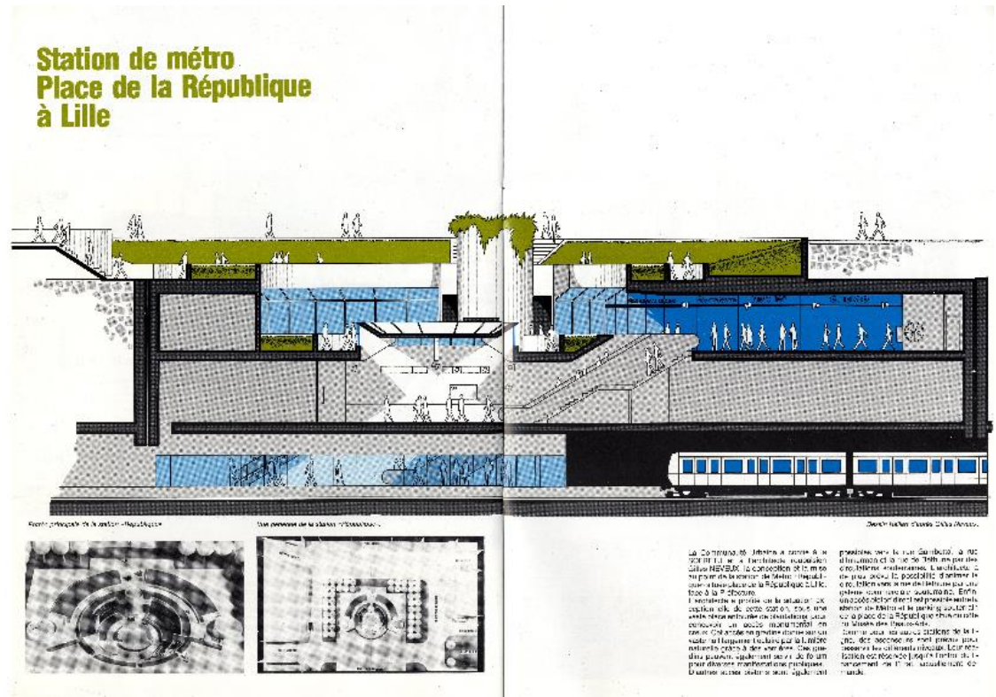
Schéma en coupe de la station République
