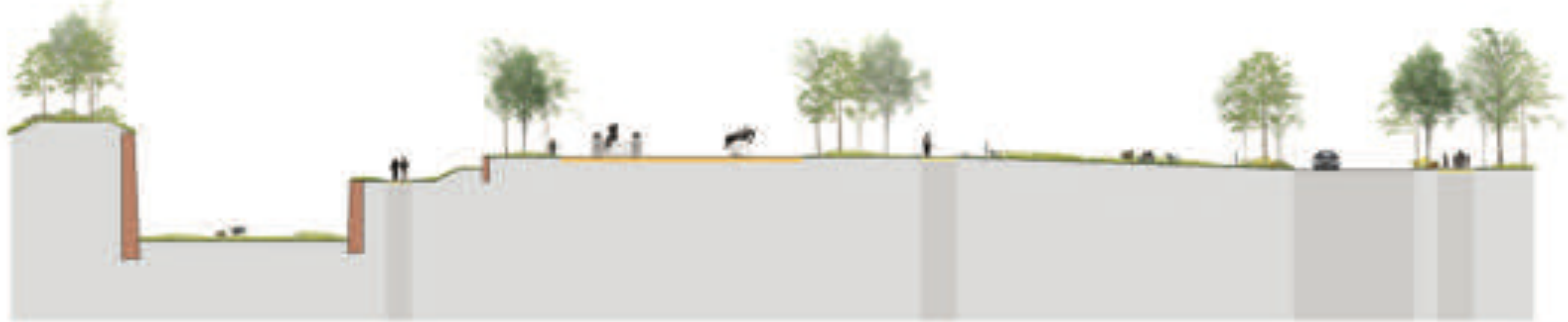
ÉCOPATURÂGE AU COEUR DES REMPARTS - COUPE GG'- 1/200e
