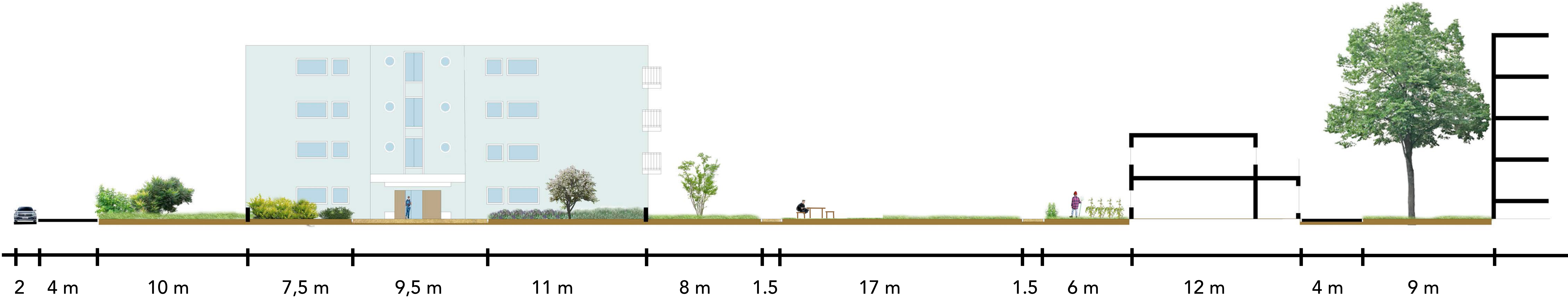
Différents seuil de collectif : jardin et frontage Coupe AA'
