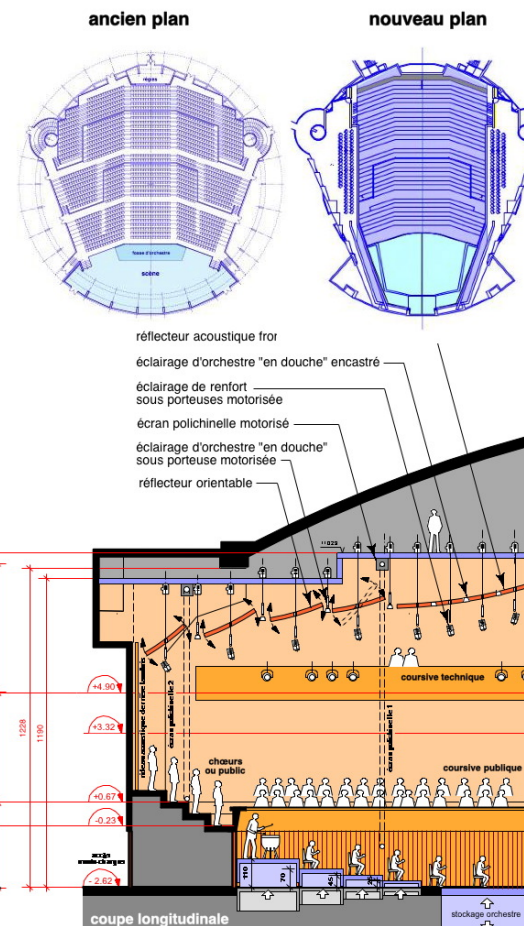
Etudes d'avant-projet de la conque acoustique
